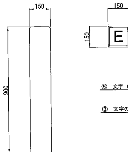
アース標 (150×150×900)
