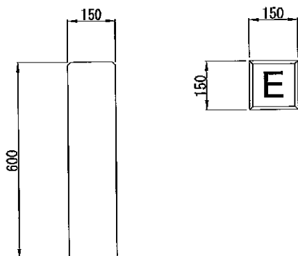
アース標 (150×150×600)
